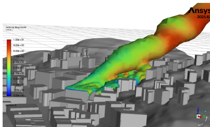
Obr. 5 Šírenie dymu Fig. 5 Smoke dissipation
