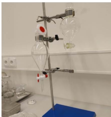
Obr. 2 Laboratórny stojan so separačným lievikom Obr. 2 Laboratory stand with a separatory funnel
