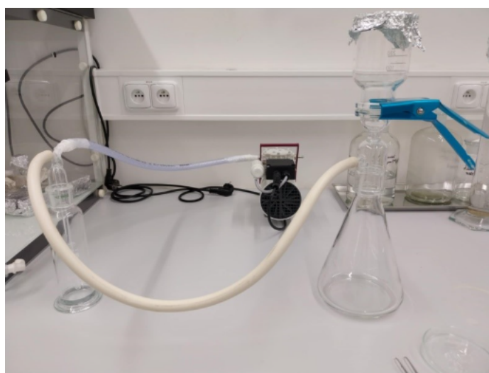
Obr. 1 Vákuová filtračná zostava Obr.1 Vacuum filtration setup
