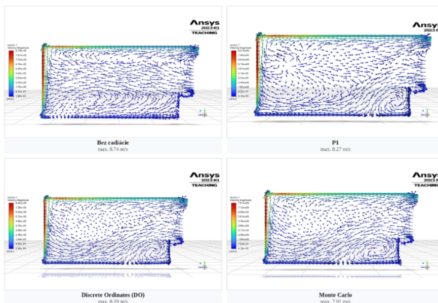
Obr. 6 Porovnanie prúdenia vzduchu (Zdroj: vlastné spracovanie) Fig. 6 Comparison of airflow (Source: own elaboration)
