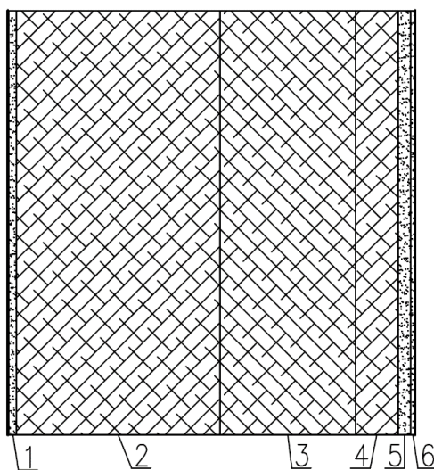
Obr. 4 Skladba obvodovej steny: OS D_I.-Z
