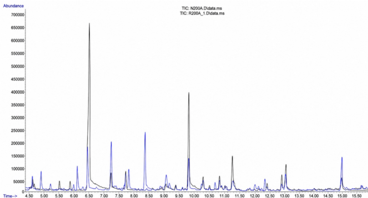
Obr. 7 Porovnanie chromatogramov prchavých produktov pri 200 °C; modrá krivka - ošetrená vzorka, čierna krivka - neošetrená vzorka
