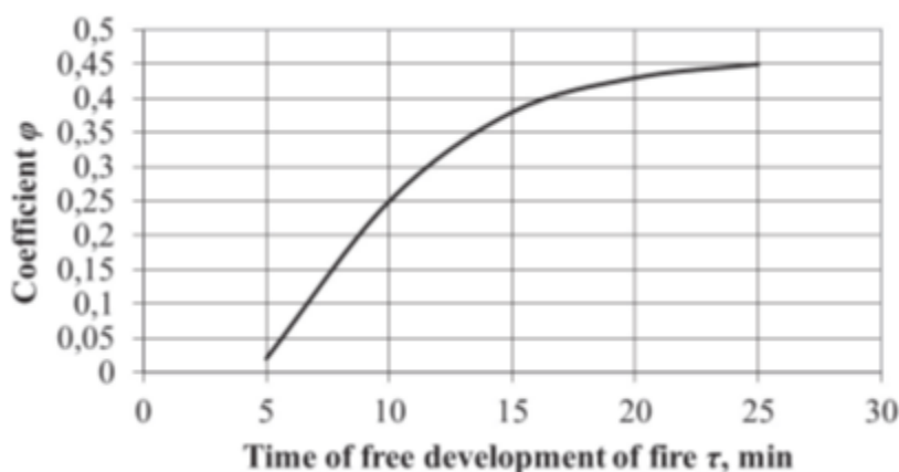
Obr. 3 Vplyv trvania voľného vývoja ohňa na hodnotu koeficientu \phi , ktorý zohľadňuje podiel tepelného toku prechádzajúceho do obvodových konštrukcií (Hulida et al., 2019)
