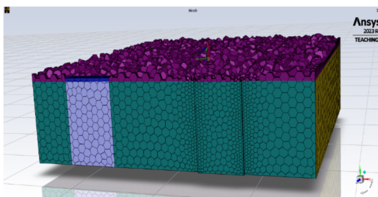
Obr. 3 Vizualizácia výpočtovej siete (Zdroj: vlastné spracovanie)
