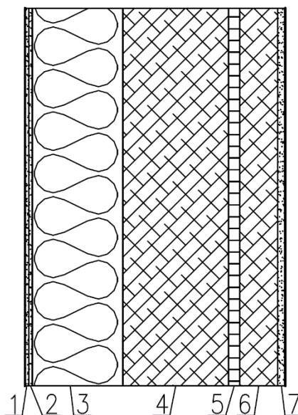
Obr. 5 Skladba obvodovej steny: OS D_III.-Z
