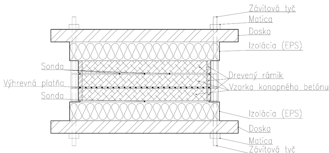
Obr. 3 Rez zostavenej meracej aparatury pre meranie tepelno-technických vlastností properties of hempcrete konopného betónu
