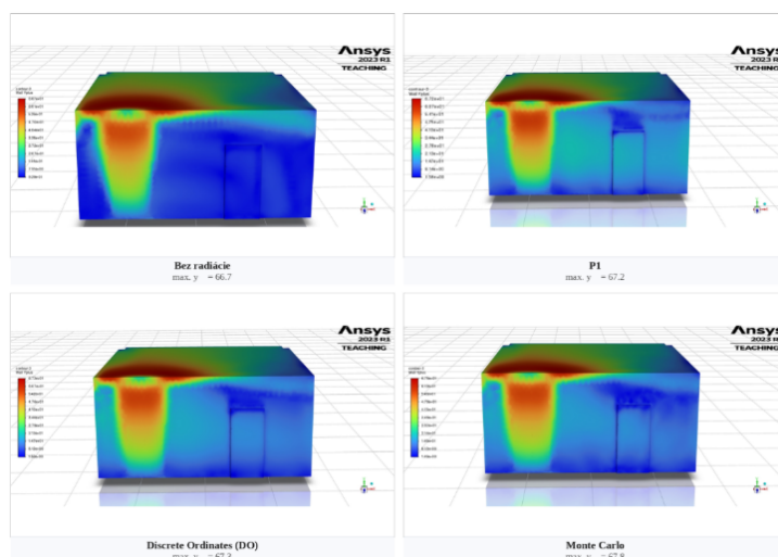
Obr. 7 Porovnanie parametra y^+ (Zdroj: vlastné spracovanie) Fig. 7 Comparison of the y^+ parameter (Source: own elaboration)
