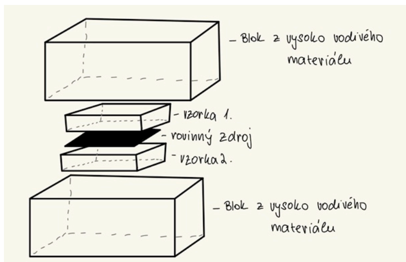
Obr. 2 Popis schémy prístroja Hot Disk, ktorý bol použitý pri metóde EDPS Fig. 2 Description of the Hot Disk device diagram, which was used in the EDPS method
