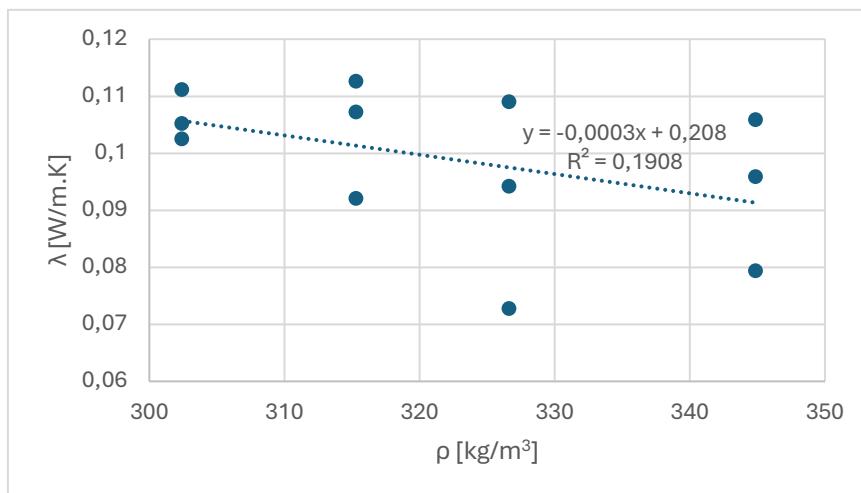
Graf 1 Vzťah hustoty a súčiniteľa tepelnej vodivosti Chart 1 Relationship between density and thermal conductivity coefficient
