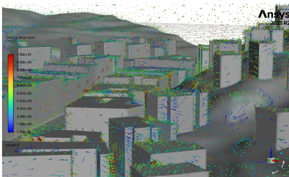
Obr. 8 Zobrazenie smeru prúdenia pomocou vektorov Fig. 8 Fluid Direction Displayed by Vectors
