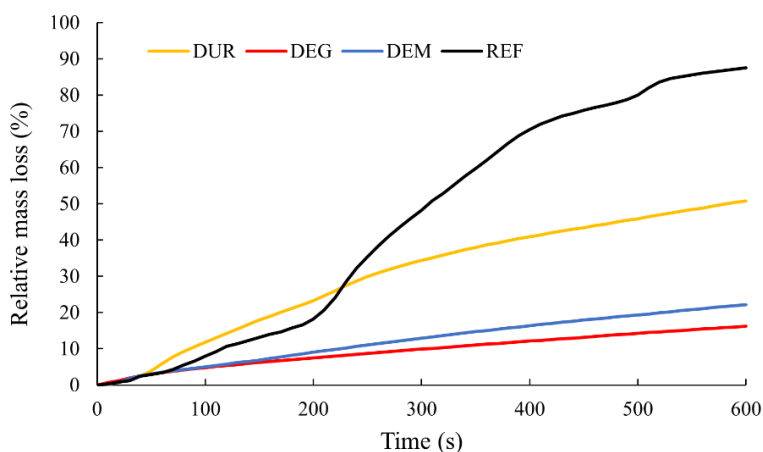
Obr. 7 Relatívna strata hmotnosti vzoriek ošetrovaných s NEODUR Fast Track Fig. 7 Relative mass loss of samples treated with NEODUR Fast Track
