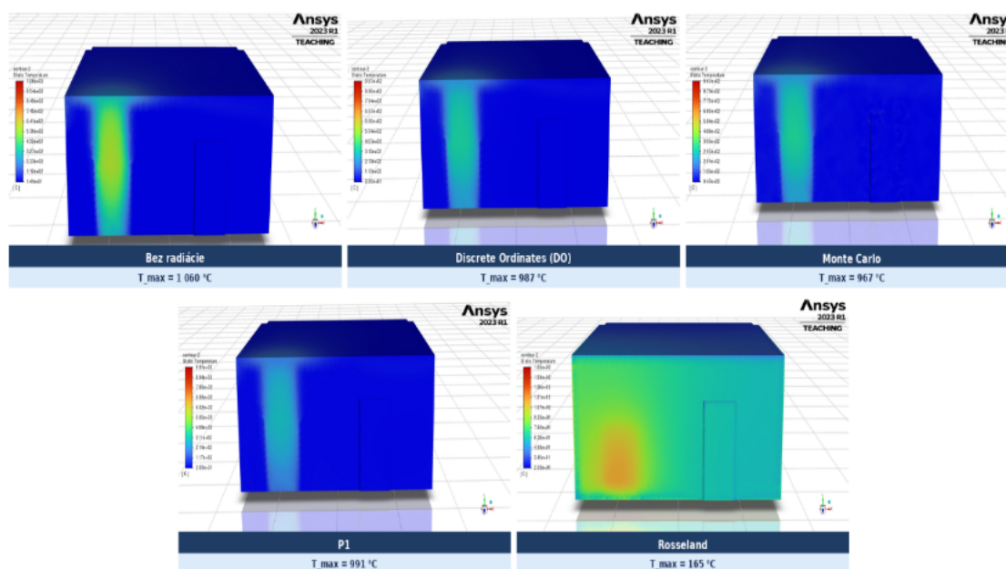
Obr. 4 Porovnanie radiačných modelov - statická teplota (Zdroj: vlastné spracovanie)
