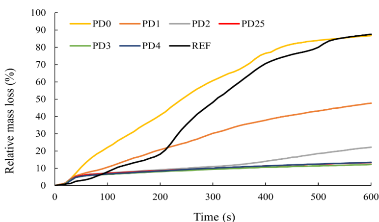
Obr. 9 Hmotnostné úbytky pri rozdielnych množstvách EG Fig. 9 Mass loss at different amounts of EG.
