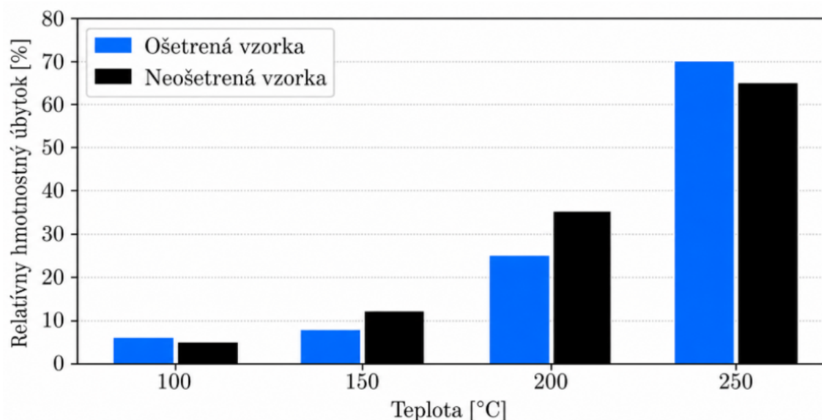
Obr. 6 Priemerné relatívne hmotnostné úbytky CLT vzoriek
