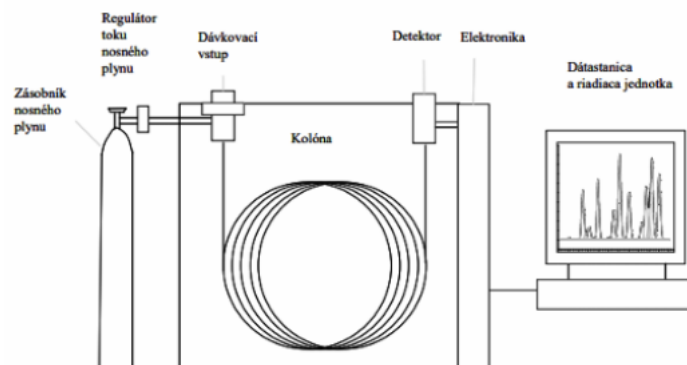
Obr. 1 Schéma plynového chromatografu (Labuda et al. 2014)
