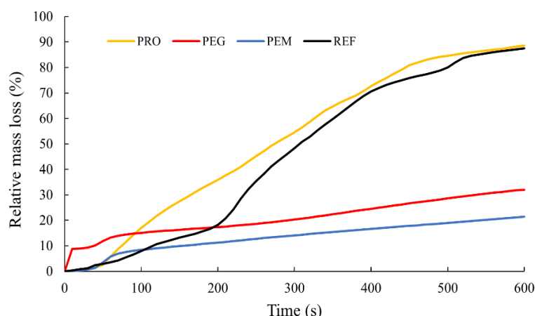
Obr. 6 Relatívna strata hmotnosti vzoriek ošetrovaných s NEOPROOF Polyurea R Fig. 6 Relative mass loss of samples treated with NEOPROOF Polyurea R
