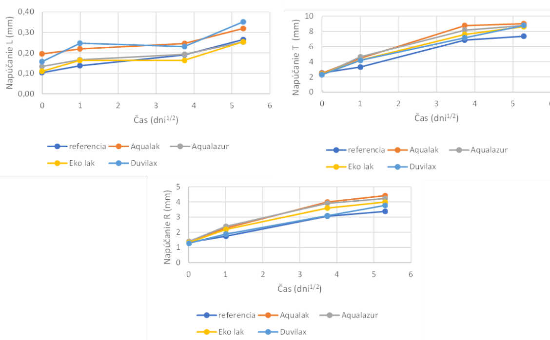
Graf 2 Napúčania v konkrétnych anatomických smeroch v čase. Fig. 2 Swelling in specific anatomical directions over time
