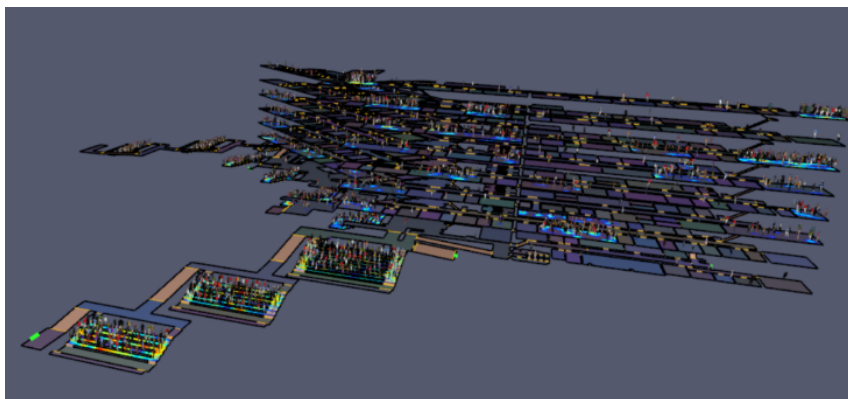
Obr. 2 Obsadenosť osôb v budove TUZVO (Pathfinder) (Zdroj: Vlastné spracovanie 2026)
