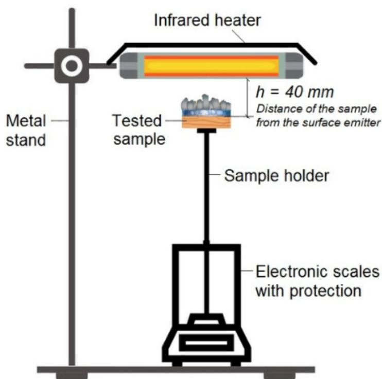
Obr. 5 Aparatúra použitá k termickému zaťažaniu (Jurczyková et al. 2024)
