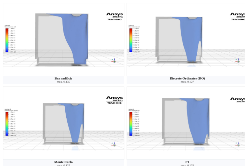
Obr. 5 Porovnanie koncentrácie CO 2 (Zdroj: vlastné spracovanie) Fig. 5 Comparison of CO 2 concentration (Source: own elaboration)
